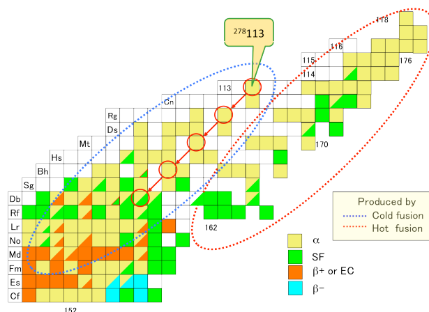
図 2.1.21: 超重核領域の核図表。
